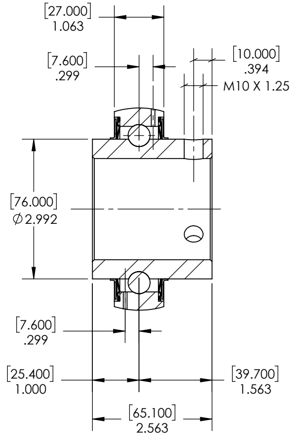
SECTION A-A
